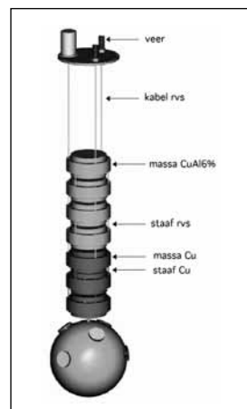
Afb. 8. De bol met zijn zeven trillingsdempers.
